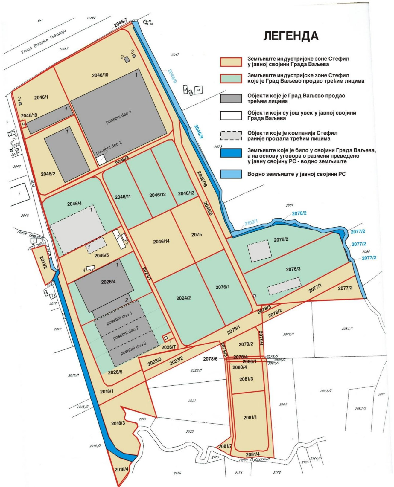
Сл.3 План површина са власничком структуром
